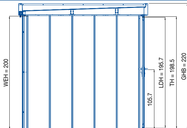
Zahradní domky na nářadí Juno s plochou střechou – pohled z boku
