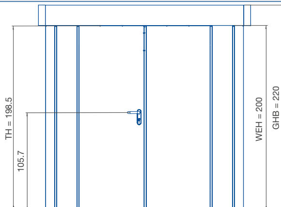
Zahradní domky na nářadí Juno s plochou střechou, dvoukřídlé – pohled zepředu
