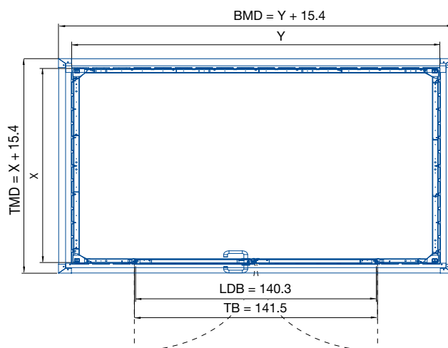
Dvoukřídlé dveře pro zahradní domky na nářadí Juno s plochou střechou
